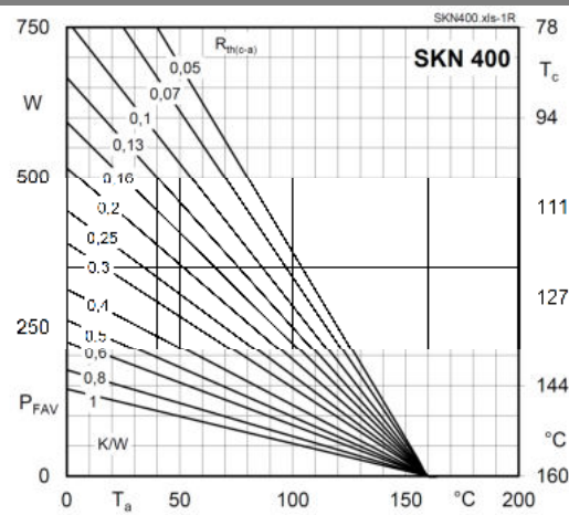
Fig. 1R Power dissipation vs. ambient temperature
